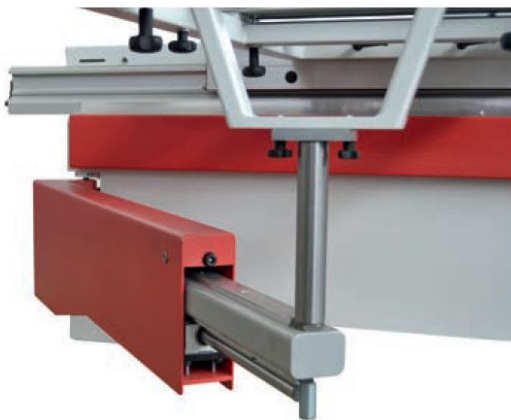
Drapeau avec manchons à billes à recirculation
